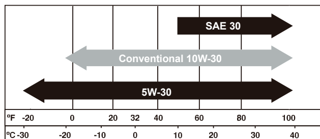
Figura 25 – Aceite recomendado
